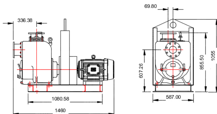
I-4 ALLPRIME Motor Elétrico 25Cv
