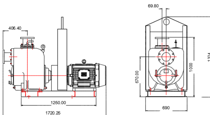
I-6 ALLPRIME Motor Elétrico 50Cv
