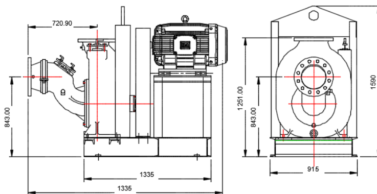
S-10ALLPRIME Motor Elétrico 100Cv
